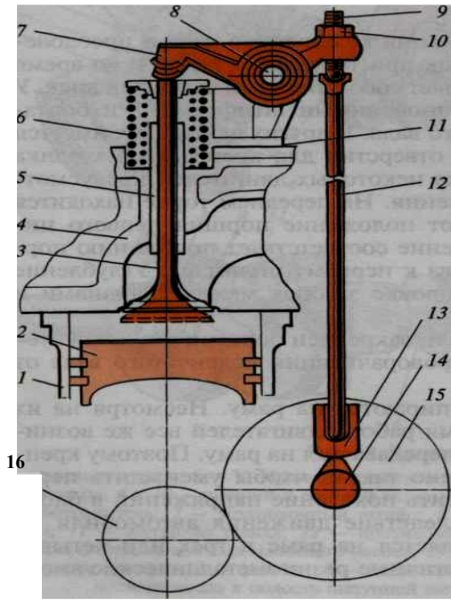
Рис.3 Схема
