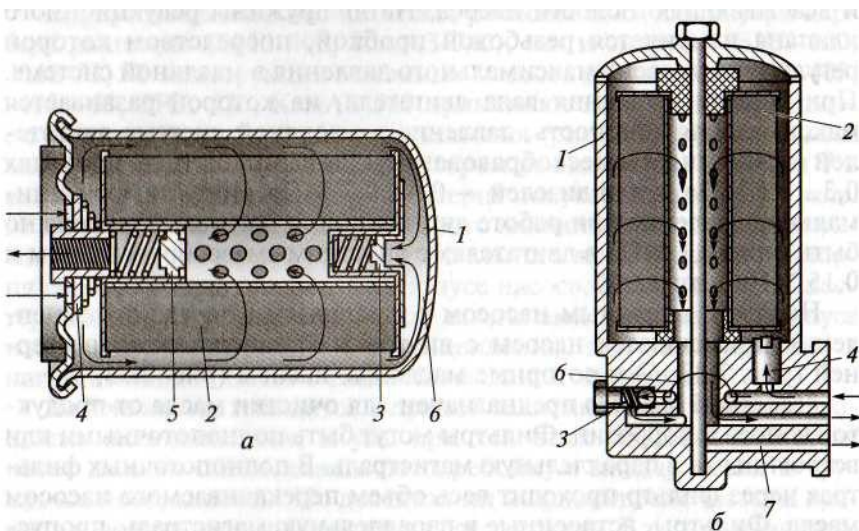
Рис. 15. Неразборный (а) и разборный (б) полнопоточные объемно-адсорбирующие фильтры.
