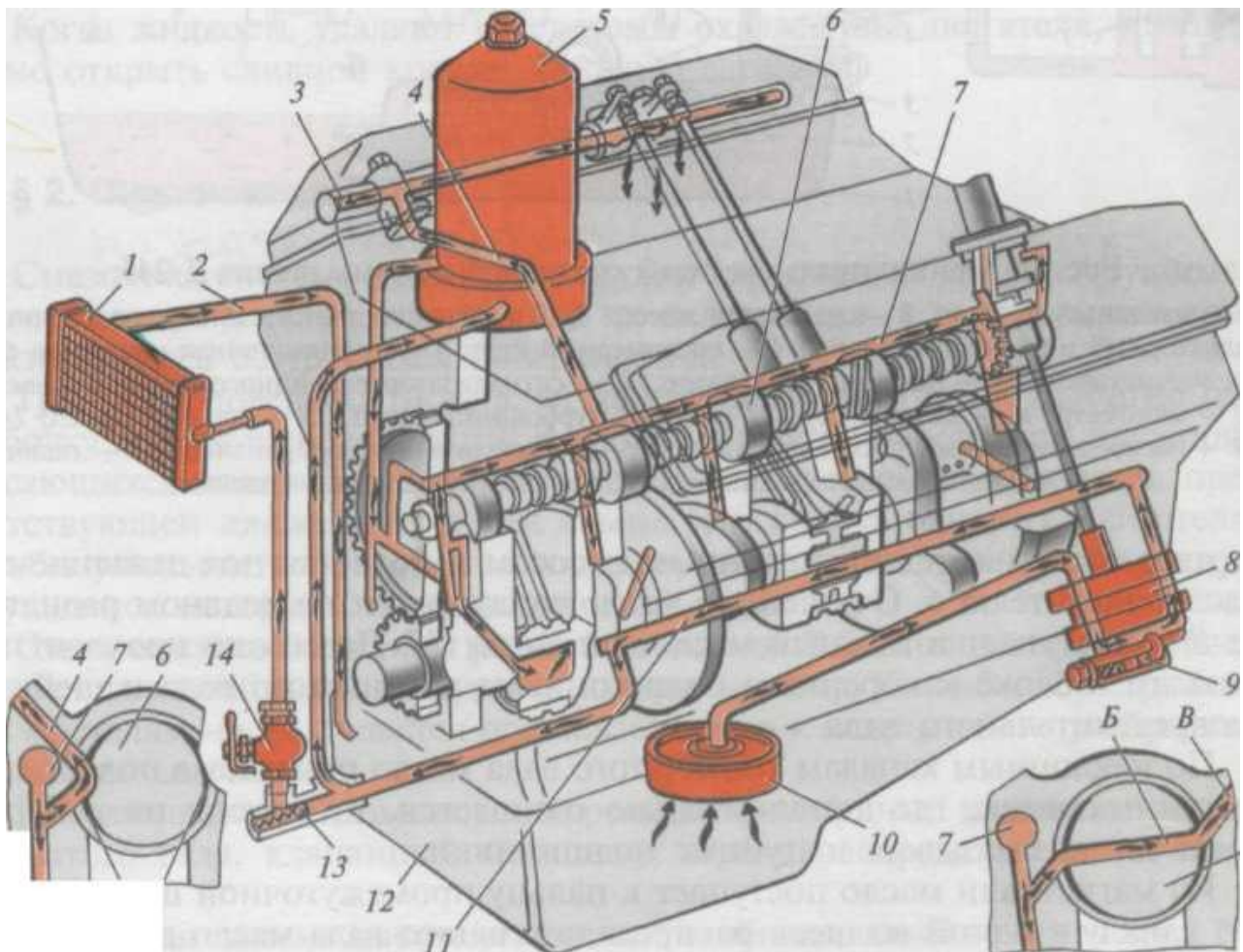
Рис.13. Смазочная система V-образного двигателя ЗМЗ-53:
