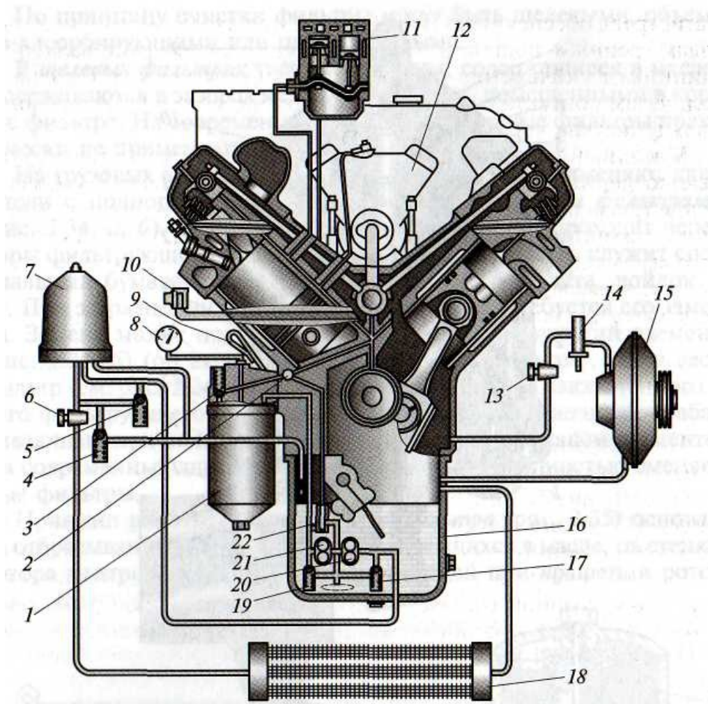
Рис. 18. Комбинированная система очистки масла двигателя КамАЗ-740:
