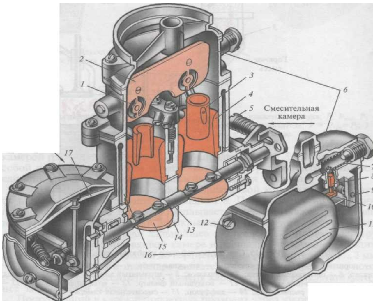
Рис. 19. Карбюратор К-135МУ:
