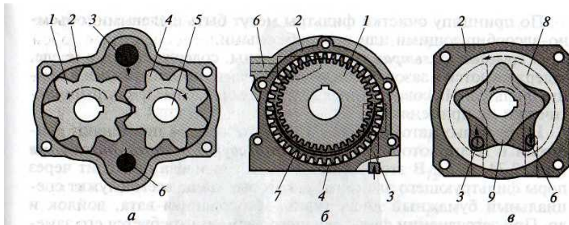
Рис. 14. Масляные насосы.
